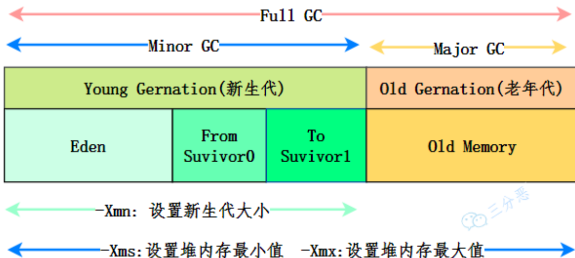
Java堆：从垃圾收集角度划分
