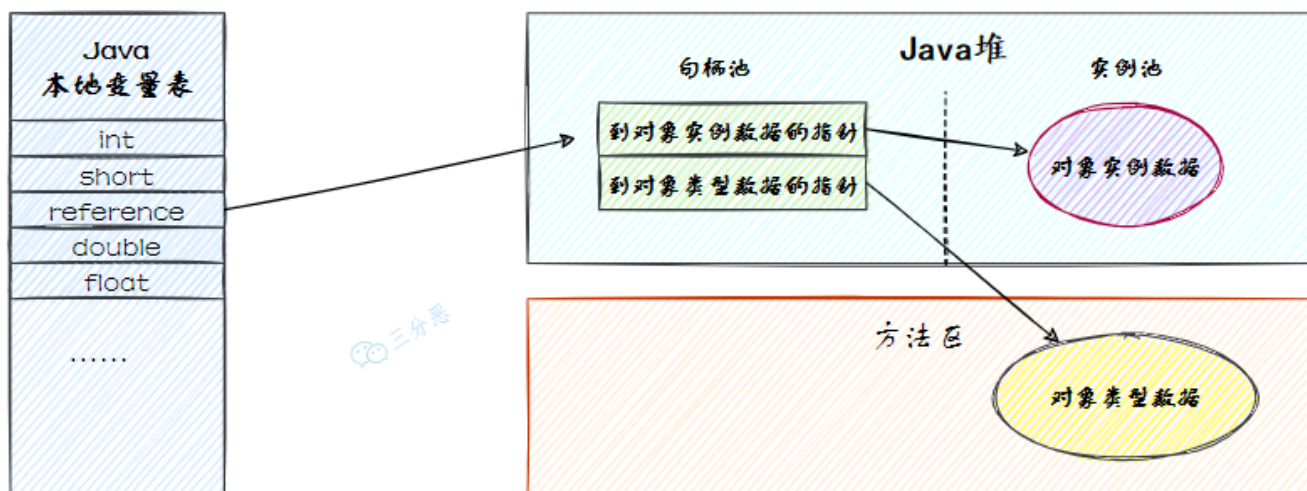
通过句柄访问对象
