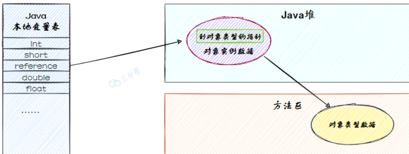
通过直接指针访问对象
